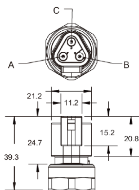
DT - Deutsch® DT04-3P
